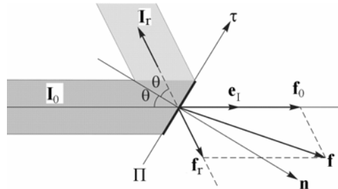
Рис. 2.5. Падающий и отраженный световые пучки и силы, действующие на пластинку П
