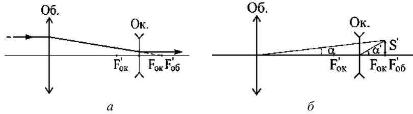
Рис. 1.15. Оптическая схема трубы Галелея (а) и к вопросу об определении углового увеличения трубы Г (б)
