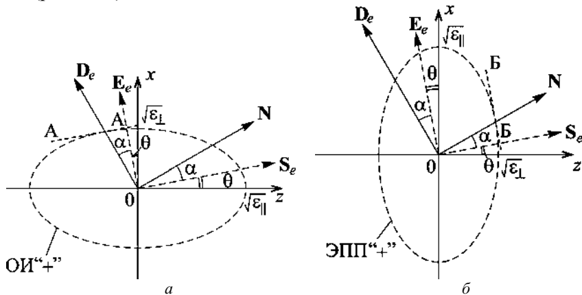
Рис. 9.5. Определение ориентации векторов E_e и S_e с помощью оптической индикатрисы (а) и эллипсоида показателя преломления (б) для положительного кристалла
