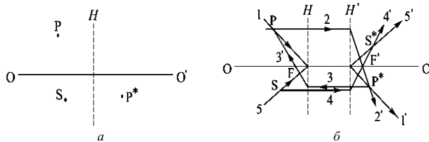
Рис.1.19. Положения главной оптической оси OO' , передней главной плоскости H , точки S и сопряженных точек P и P^* (а); построения для нахождения положения точки S^* , сопряженной с точкой S (б)
