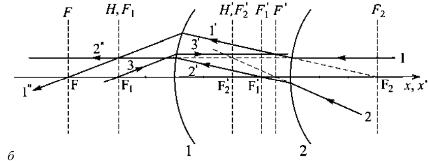
Рис.1.18. а – оптическая схема толстой выпукло-вогнутой линзы; б – ход лучей через толстую выпукло-вогнутую линзу
