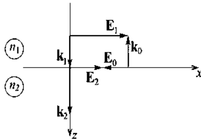
Рис. 7.5. Схема расположения векторов k 1 , k 2 , k 0 и амплитуд электрического поля в падающей, отраженной и преломленной волнах
