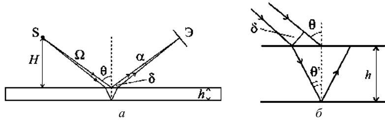
Рис. 3.13. Схема получения интерференционной картины от точечного источника S с помощью тонкой слюдяной пластинки ( a ); ход лучей в пластинке ( b )
