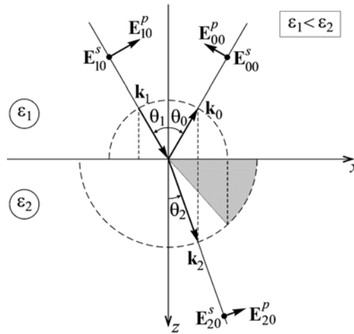
Рис.7.1. Отражение и преломление света на границе раздела двух сред с проницаемостями \varepsilon_1 < \varepsilon_2
