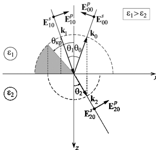
Рис.7.2. Отражение и преломление света на границе раздела двух сред с проницаемостями \varepsilon_1 > \varepsilon_2
