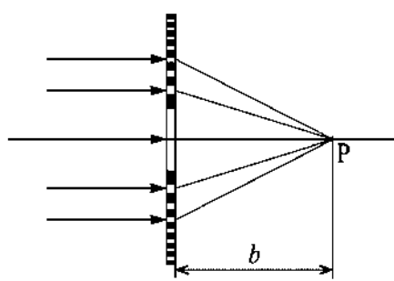
Рис. 4.19. Положение точки Р относительно зонной пластинки
