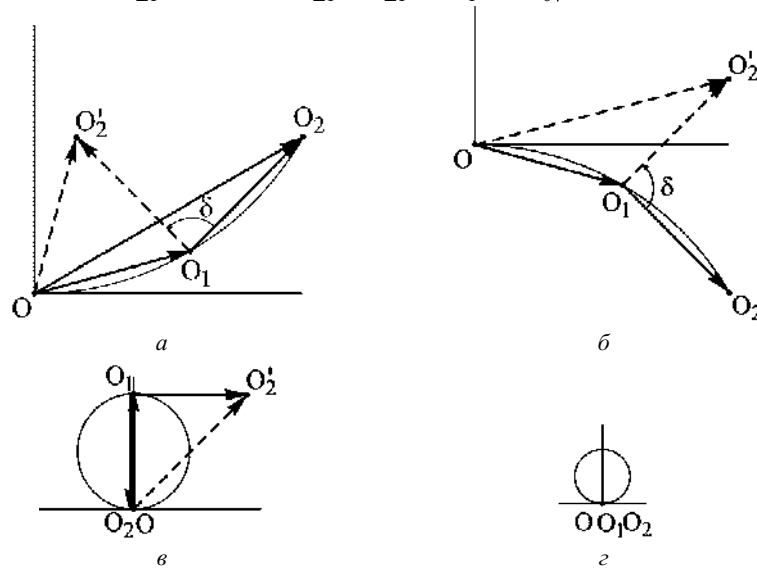
Рис. 5.7. Векторные диаграммы: для произвольного угла дифракции \varphi > 0 (а) и \varphi < 0 (б), для направлений на первый (в) и второй (г) дифракционный минимум
