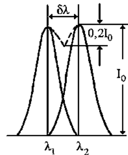
Рис. 6.2. Разрешающая способность спектрального прибора по Рэлю
