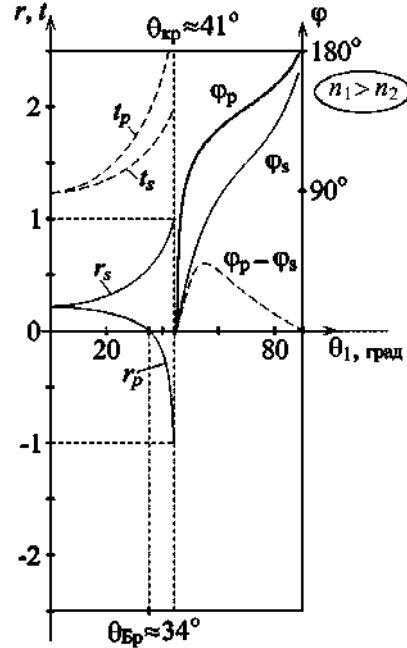
Рис.7.4. Коэффициенты отражения r и пропускания t для волн с s - и p -поляризацией в зависимости от угла падения \theta_1 на поверхность раздела двух сред ( n_1 > n_2 , n_1 = 1,5 n_2 ); \varphi_p и \varphi_s – набег фазы при полном внутреннем отражении.
