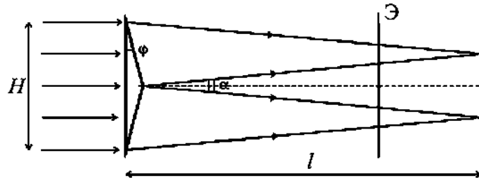
Рис. 3.10. Наблюдение интерференционной картины с помощью бипризмы
