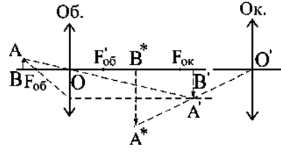
Рис. 1.17. Ход лучей в микроскопе
