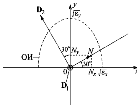
Рис.9.8. Расположение векторов \mathbf{D}_1 и \mathbf{D}_2 относительно оптической индикатрисы
