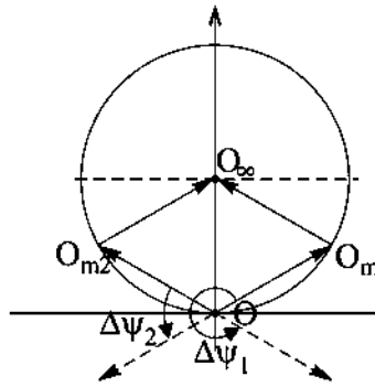
Рис.4.14. Два возможных случая направления вектора \vec{OO}_{m1} и \vec{OO}_{m2}
