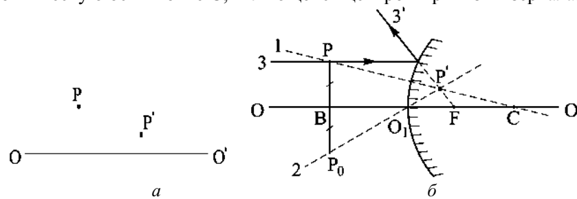
Рис. 1.10. Положения сопряженных точек Р и Р' относительно оптической оси ОО' сферического зеркала (а) и вспомогательные построения при определении положения зеркала и его фокуса (б)
