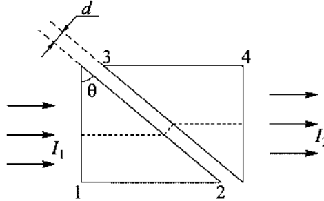
Рис. 7.8. Прохождение лазерного излучения через две прямоугольных призмы с зазором
