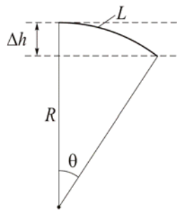
Рис. 8.3. К вопросу об изгибе луча света вблизи поверхности Земли
