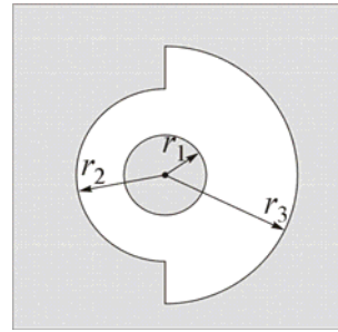
Рис. 4.8. Форма отверстия в экране
